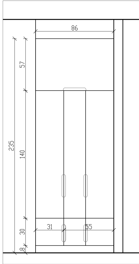
ארון - חזית קדמית
